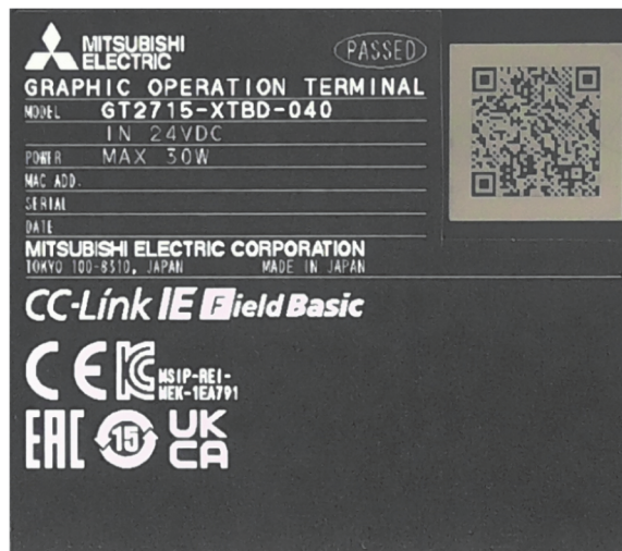
代替品の定格銘板(UL 認証マークなし)
